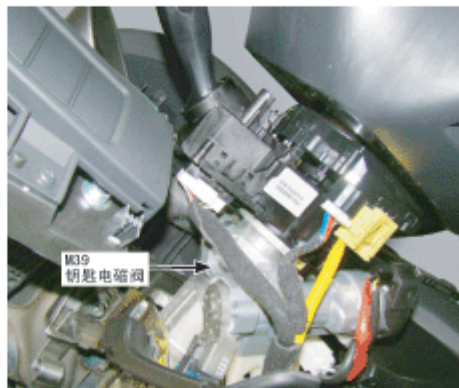
81. 转向柱
